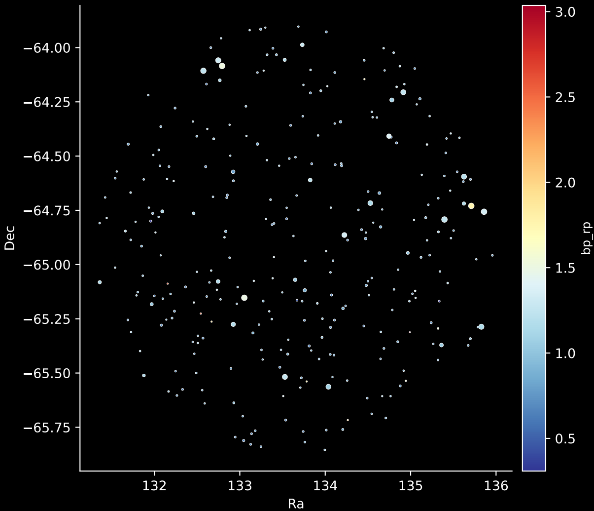
GALAH DR4 Field: [7006] Stars: 299
