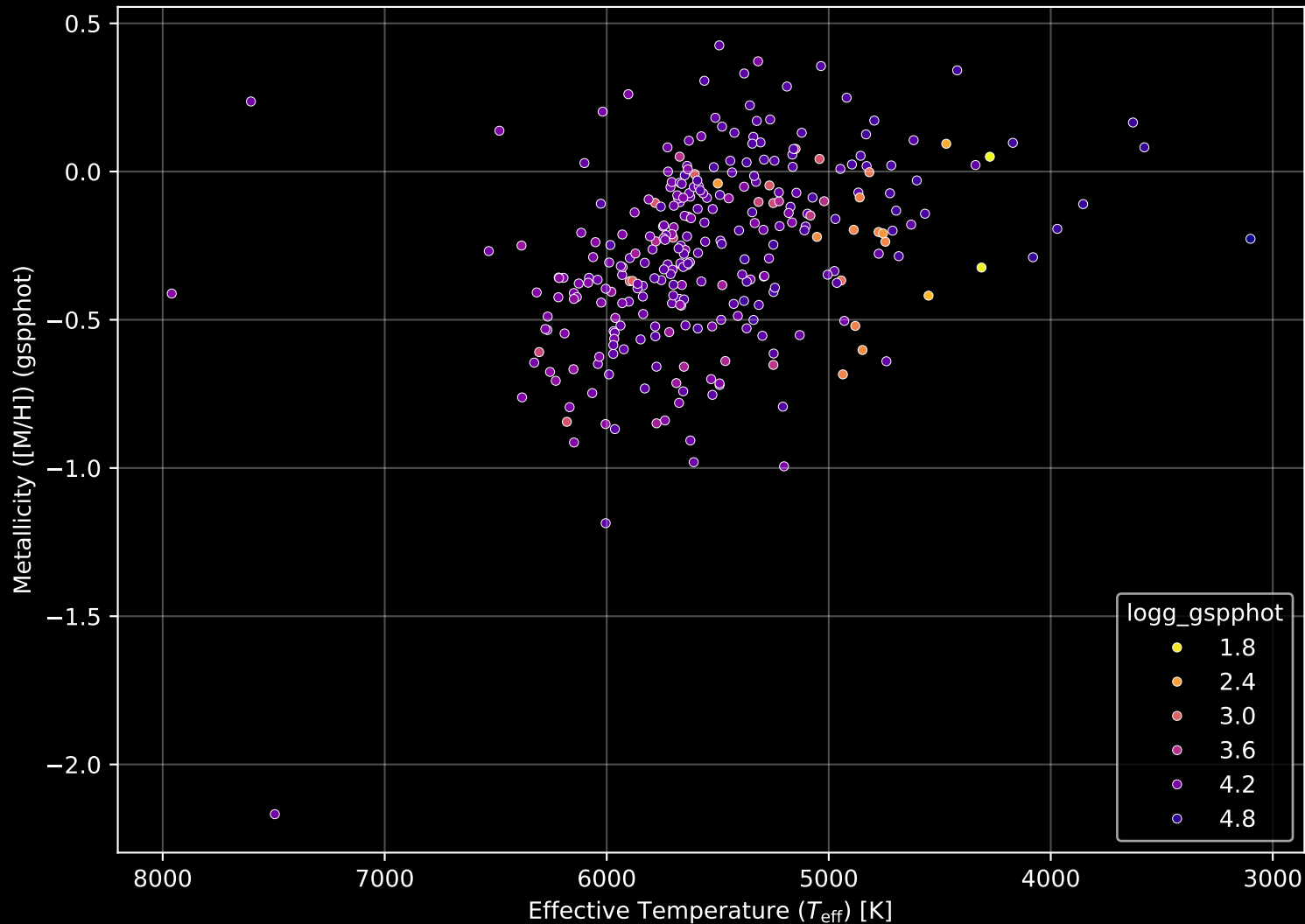
GALAH DR4 Field: [7006] Stellar Population Parameters (n= 299)
