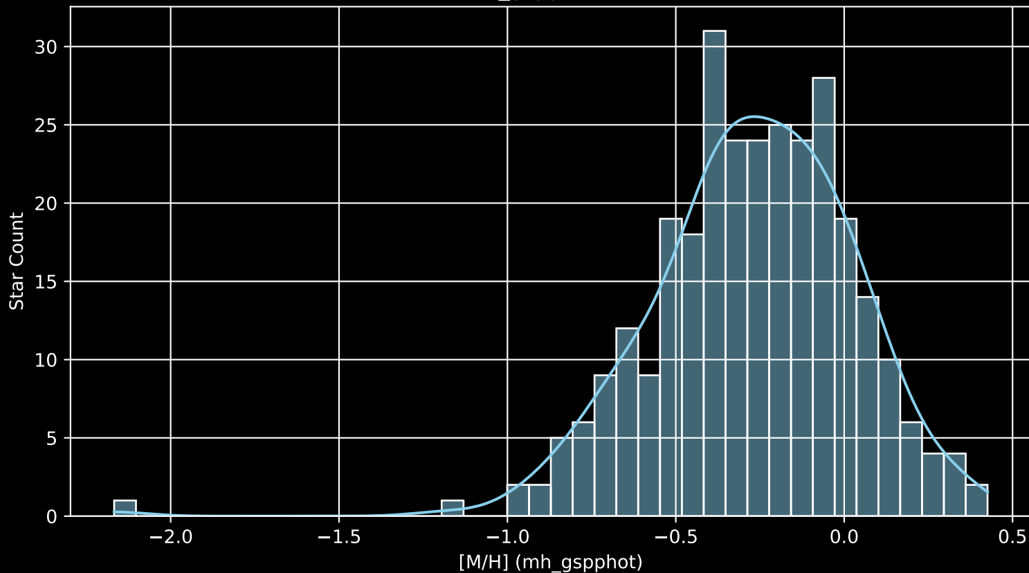
GALAH DR4 Field: [7006] [M/H] (mh_gspphot) (n= 299)
